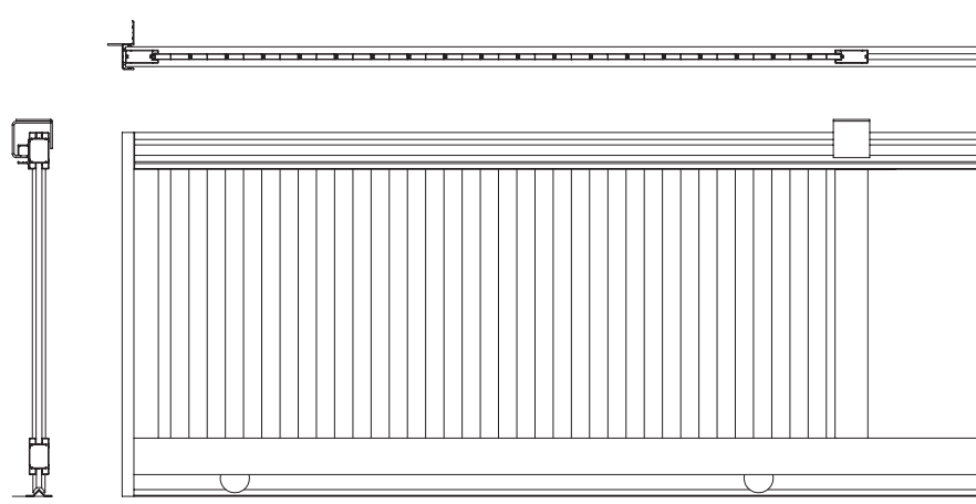
PORTAIL COULISSANT
