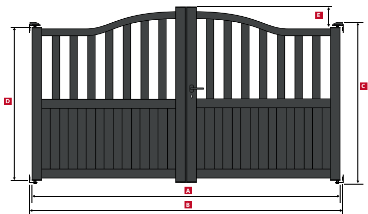
LEVANT Portail Battant / Swing gate / Drehtor
