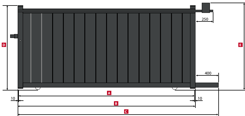
BREST Portail Coulissant / Sliding gate / Schiebetor Annexe / Appendix / Annex: 1 Tableau / Table / Tabelle: 3
