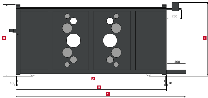
MIAMI Portail Coulissant / Sliding gate / Schiebetor Annexe / Appendix / Annex: 1 Tableau / Table / Tabelle: 3
