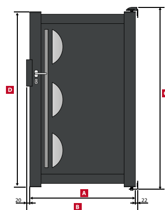
TRENTON Portillon / Side gate / Gartentür
