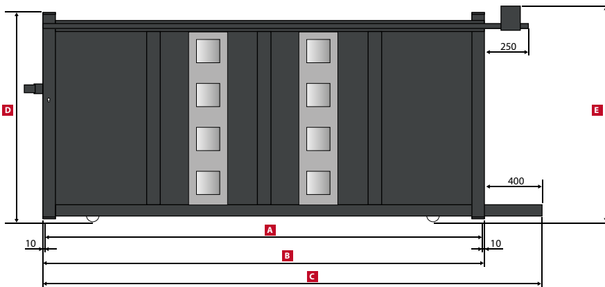
PHOENIX Portail Coulissant / Sliding gate / Schiebetor Annexe / Appendix / Annex: 1 Tableau / Table / Tabelle: 3
