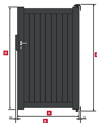
ANTILLES Portillon / Side gate / Gartentür
