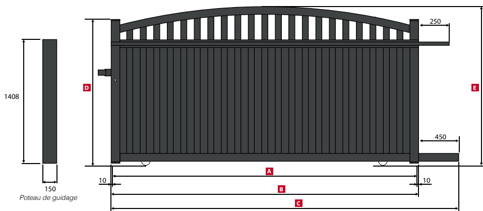
ARAL Portail Coulissant / Sliding gate / Schiebetor Annexe / Appendix / Annex: 1 Tableau / Table / Tabelle: 4
