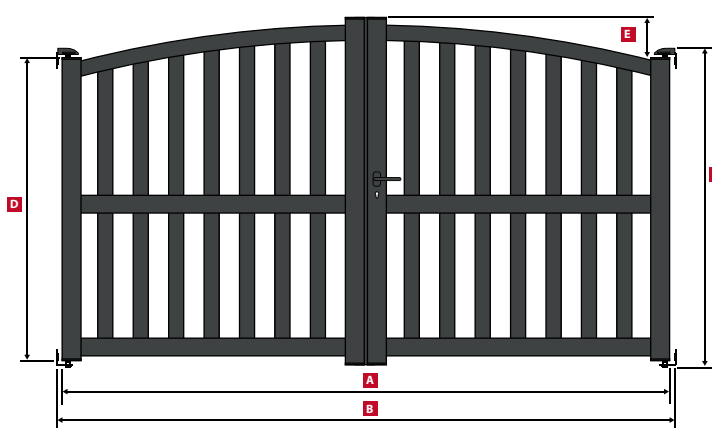
CORAIL Portail Battant / Swing gate / Drehtor
