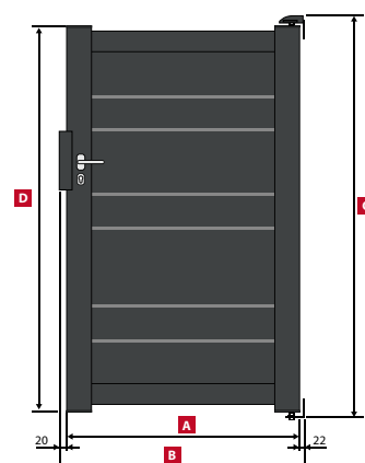
LILLE Portillon / Side gate / Gartentür Annexe / Appendix / Annex: 2 Tableau / Table / Tabelle: 2
