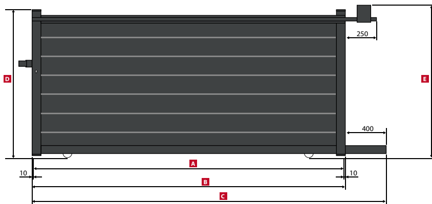
NÎMES Portail Coulissant / Sliding gate / Schiebetor Annexe / Appendix / Annex: 1 Tableau / Table / Tabelle: 3
