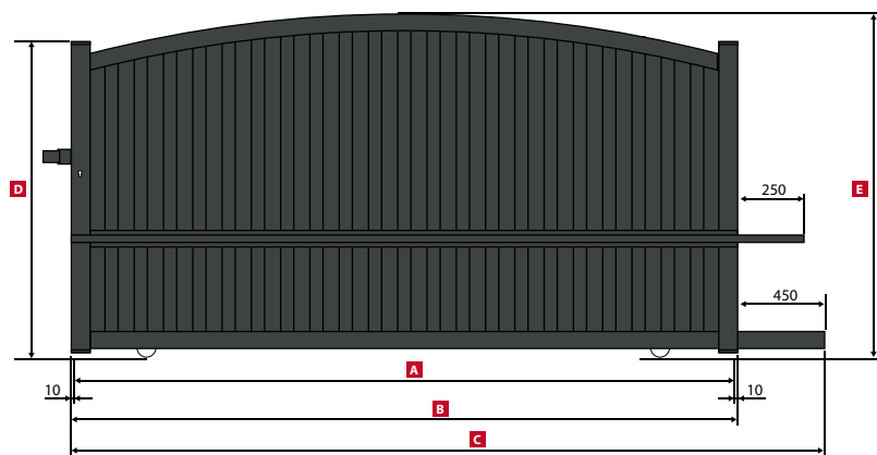
ADRIATIQUE Portail Coulissant / Sliding gate / Schiebetor
