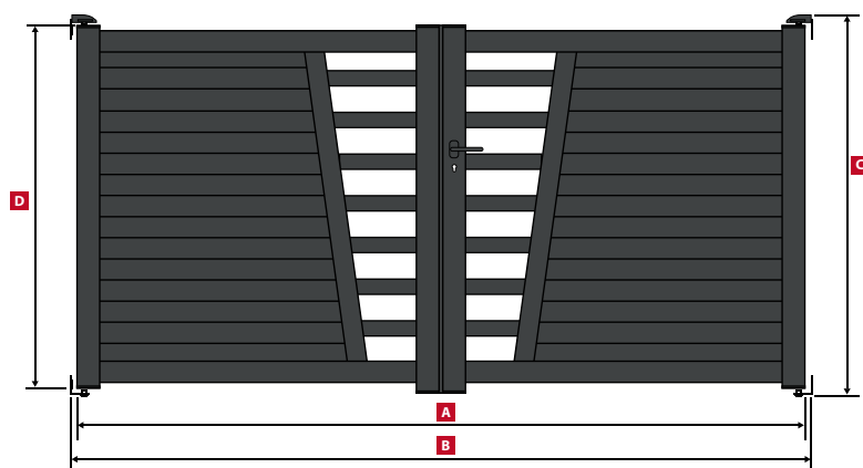
LICOLIN Portail Battant / Swing gate / Drehtor
