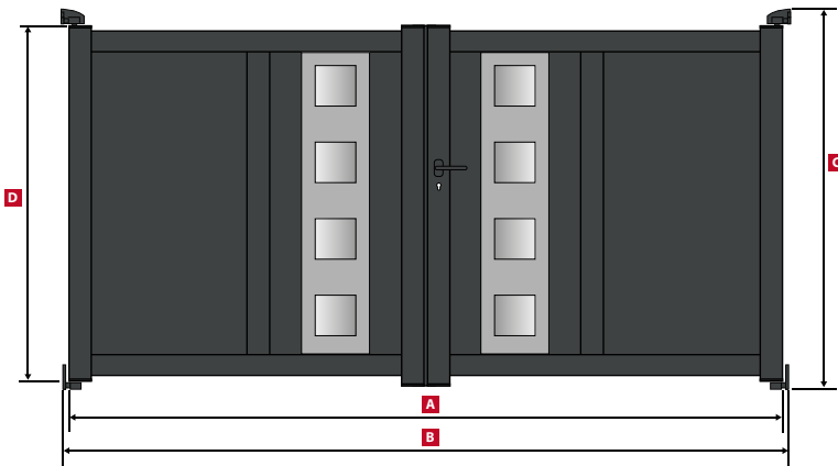
PHOENIX Portail Battant / Swing gate / Drehtor Annexe / Appendix / Annex: 1 Tableau / Table / Tabelle: 2
