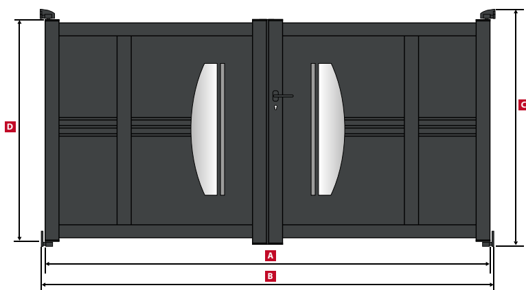
HOUSTON Portail Battant / Swing gate / Drehtor
