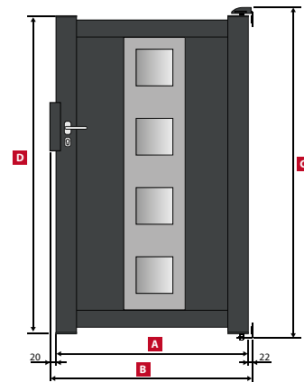
PHOENIX Portillon / Side gate / Gartentür Annexe / Appendix / Annex: 2 Tableau / Table / Tabelle: 2
