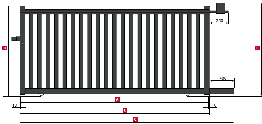
ADEN Portail Coulissant / Sliding gate / Schiebetor
