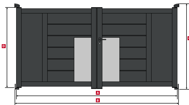
BOSTON Portail Battant / Swing gate / Drehtor
