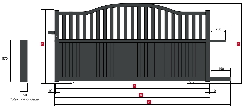
LEVANT Portail Coulissant / Sliding gate / Schiebetor
