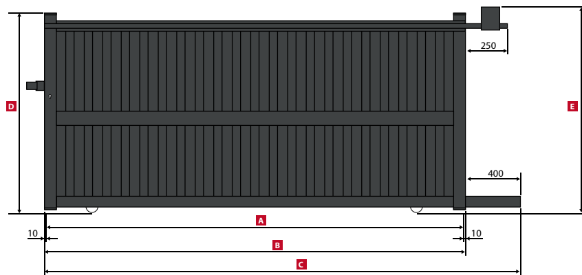
MELVILLE Portail Coulissant / Sliding gate / Schiebetor
