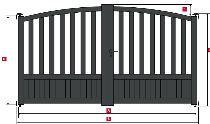
PHILIPPINES Portail Battant / Swing gate / Drehtor
