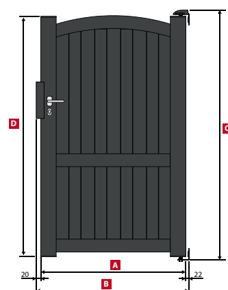
ADRIATIQUE Portillon / Side gate / Gartentür
