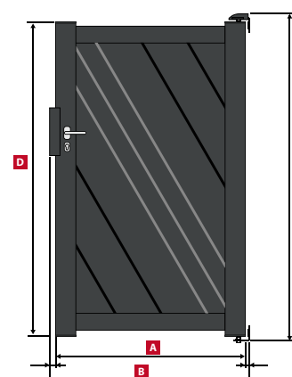
ORLÉANS Portillon / Side gate / Gartentür
