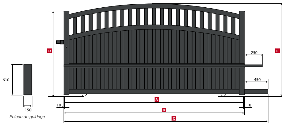
CAMOTES Portail Couissant / Sliding gate / Schiebetor
