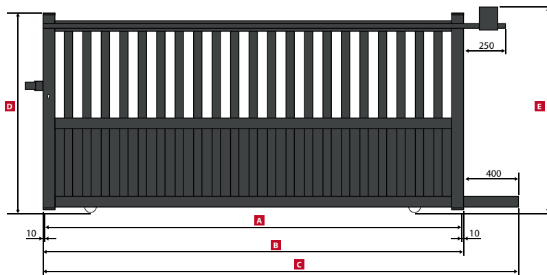
KINLEY Portail Couissant / Sliding gate / Schiebetor Annexe / Appendix / Annex: 1 Tableau / Table / Tabelle: 3
