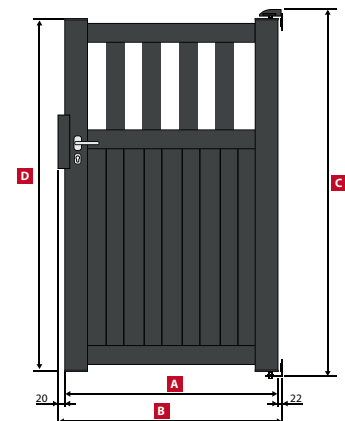
WEDEL Portillon / Side gate / Gartentür Annexe / Appendix / Annex: 2 Tableau / Table / Tabelle: 2
