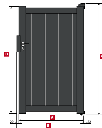
NICE Portillon / Side gate / Gartentür Annexe / Appendix / Annex: 2 Tableau / Table / Tabelle: 2
