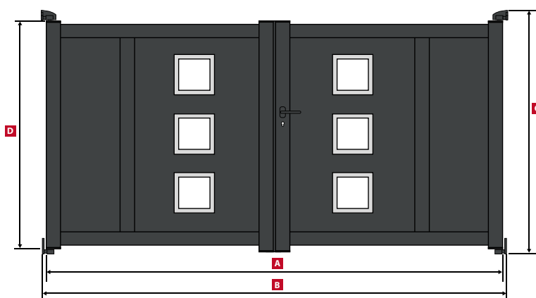
DAYTON Portail Battant / Swing gate / Drehtor
