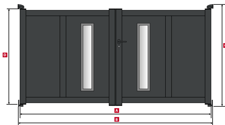
DALLAS Portail Battant / Swing gate / Drehtor
