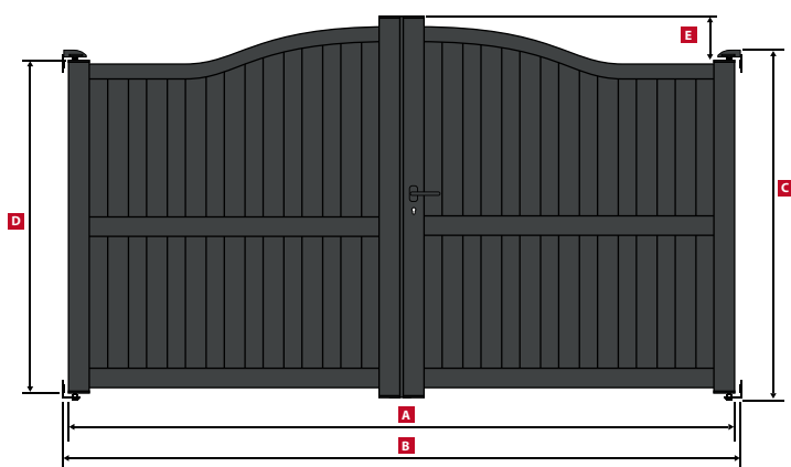
MARMARA Portail Battant / Swing gate / Drehtor
